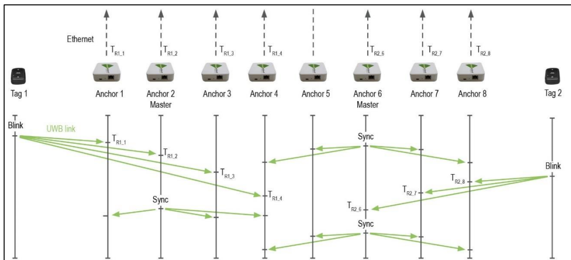
22. ábra - TDoA távolságmérés és időszinkronizáció több Anchor csoport esetében [29]
