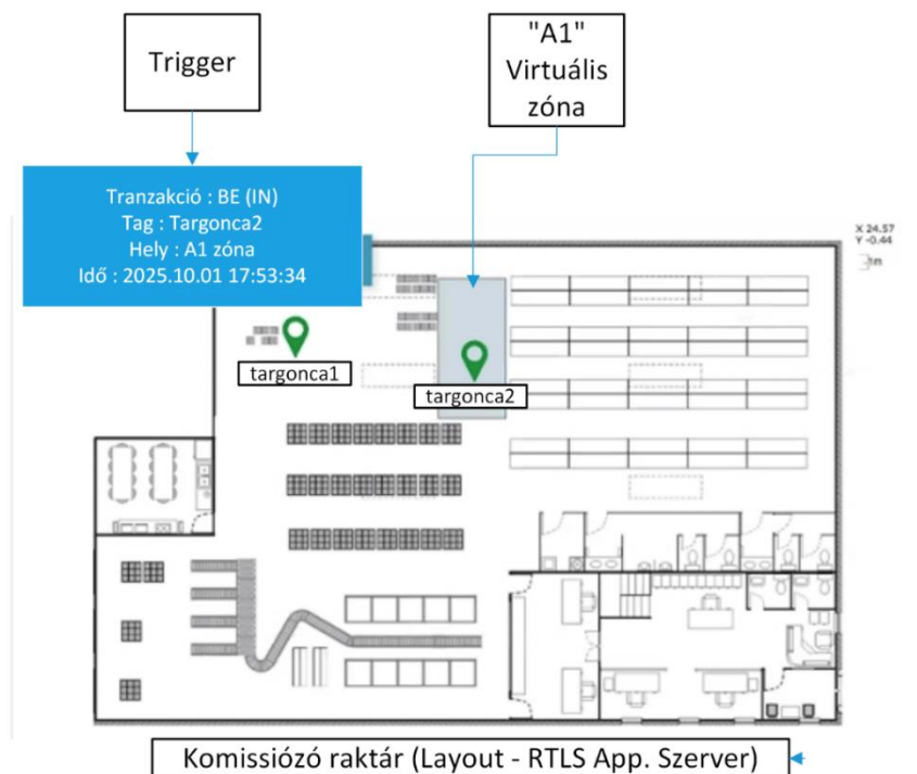
41. ábra – Virtuális zóna és trigger az RTLS applikációs szerver raktári layout-ján
