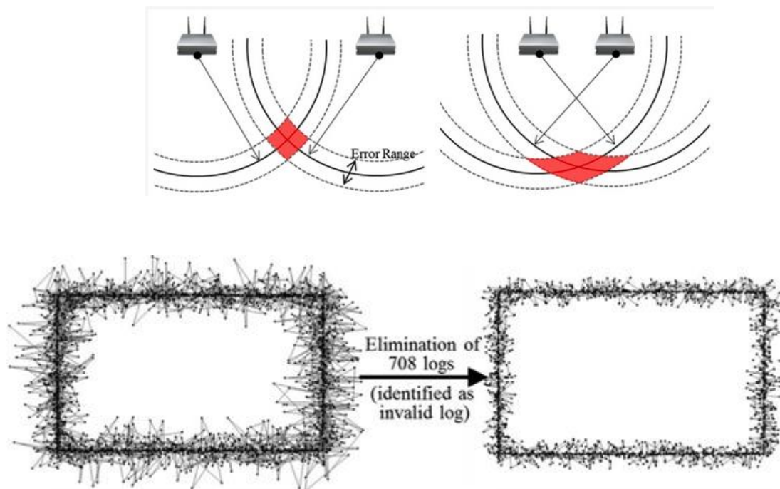
13. ábra - Nem pontos távolságmérés esetében algoritmus vagy szűrő segítségével becsülhető meg a pont pozíciója
