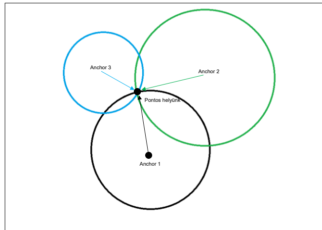
12. ábra – Helymeghatározás síkban, 3 darab Anchor segítségével, ideális esetben
