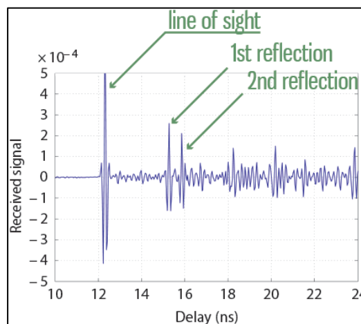
15. ábra - UWB impulzusjel visszaverődései az Anchornál
