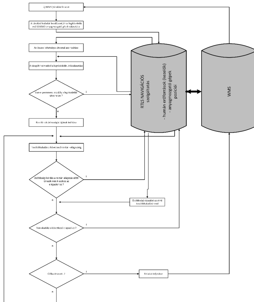
58. ábra - tárolási művelet algoritmus a WMS + RTLS raktári menedzsment modellben
