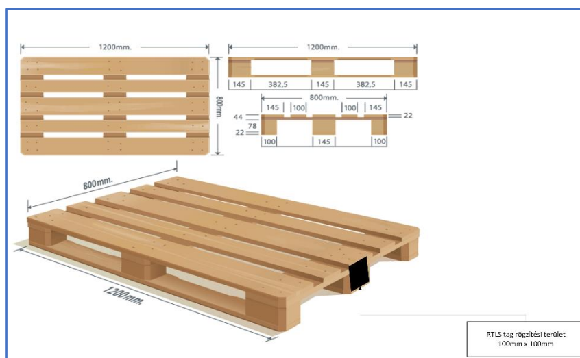
35. ábra - RTLS tag általános rögzítési pozíciója EUR raklap esetében
