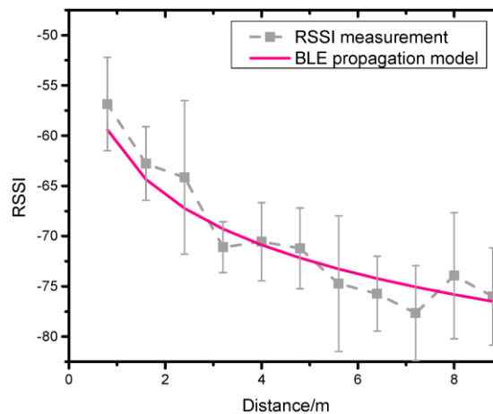
24. ábra - BLE-RSSI technológia mérési pontatlansága [25], két mérendő pont távolsága között nagy amplitúdójú „ugrások” érzékelhetők
