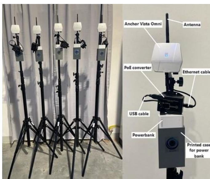
51. ábra - Pilot RTLS rendszer hardver elemei [77]
