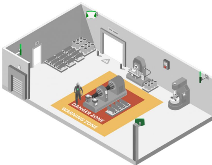
44. ábra - Veszélyzónák létrehozása virtuális zóna segítségével
