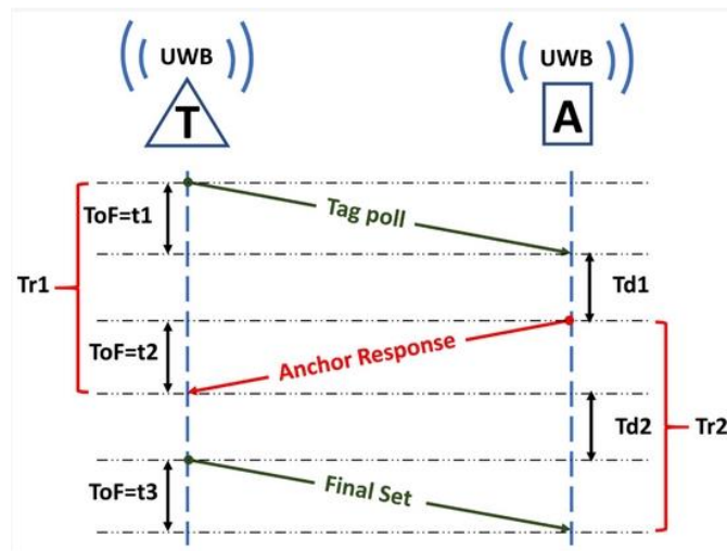
21. ábra - UWB szabványú (A) Anchor és (T) RTLS Tag közötti távolságmérés – TWR protokollal [28]
